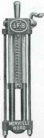
manomètre clef ouverte réglage du zéro
