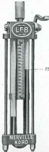
manomètre raccordé pression 75 mm. d'eau
